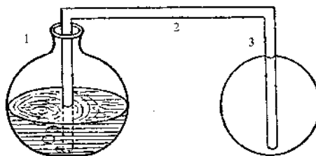
Рис. 6.38. Термоскоп Филона
