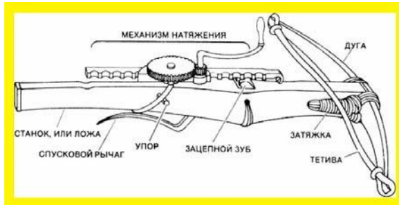
Рис. 6.24. Французский вариант зарядного и спускового устройства
