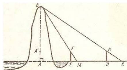
Рис. 3.12. Измерительный шест
