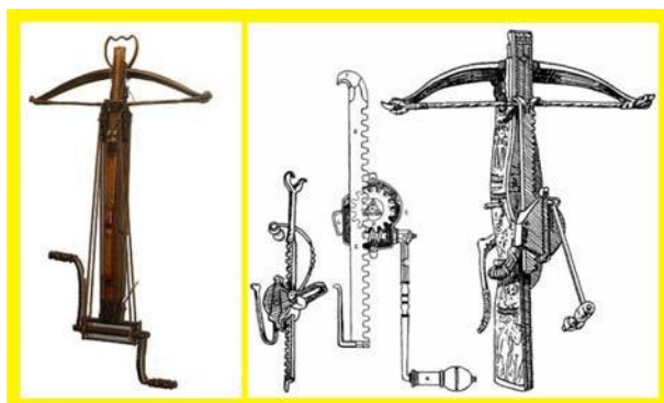
Рис. 6.21. Способы взведения арбалета воротом и рейкой с шестернёй
